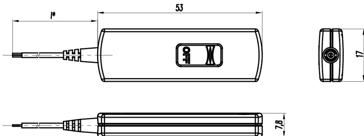
Габаритные размеры переключателя
