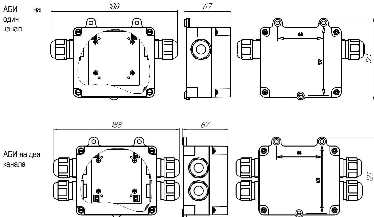
Рис.1 – Установочные размеры одноканального и двухканального АБИ.
