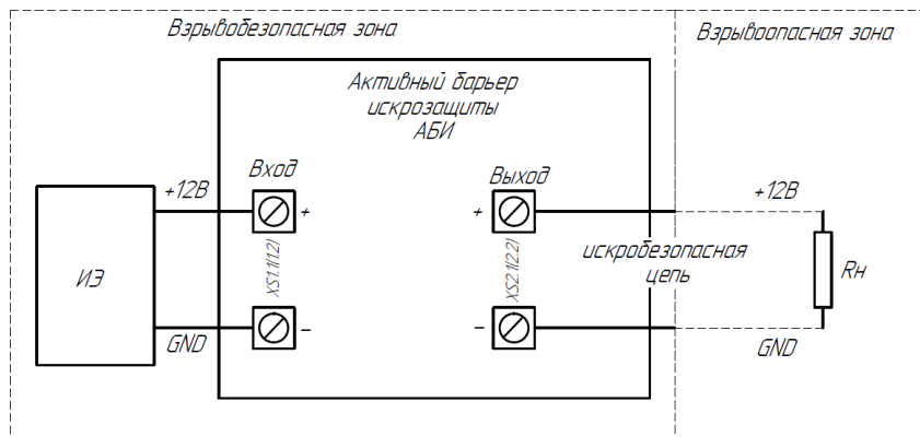
Рис.2 – Клеммные соединения барьера АБИ (один канал)
