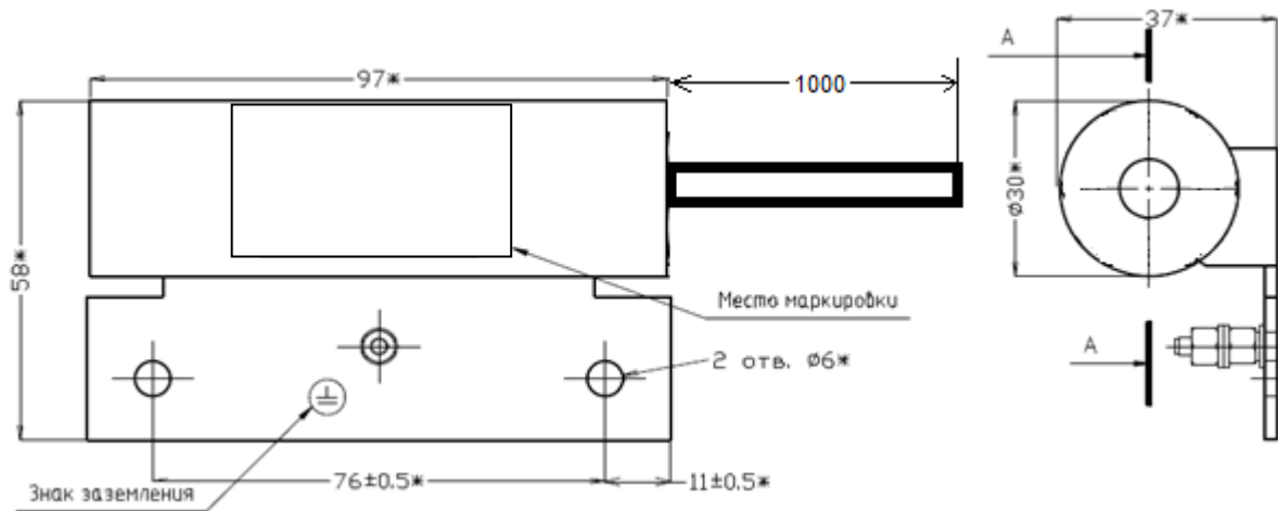
Рис. 6 конструкция датчиков Ex IO 102 «ЛЁД» с постоянно присоединенным кабелем.
