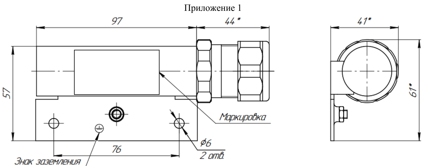
Рис.1 Габаритные и установочные размеры исполнительного блока Ex ИО 102 «ЛЁД»
