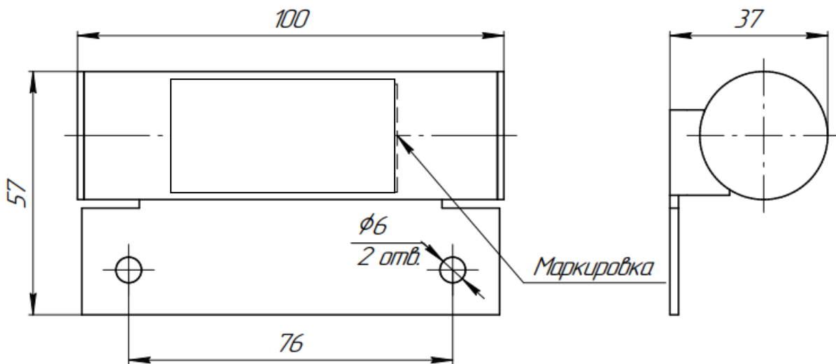
Рис.3 Габаритные и установочные размеры задающего блока Ех ИО 102 «ЛЁД»
