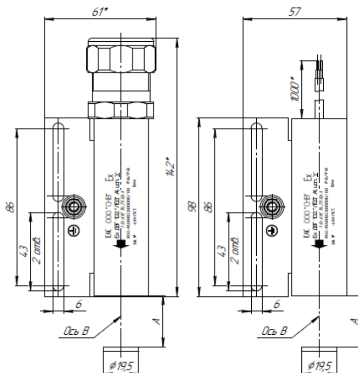
Рис.7. конструкция датчиков Ex IO 102 «ЛЁД» с торцевой рабочей зоной, постоянно присоединенным кабелем или кабельным вводом и креплением к поверхности на кронштейне.
