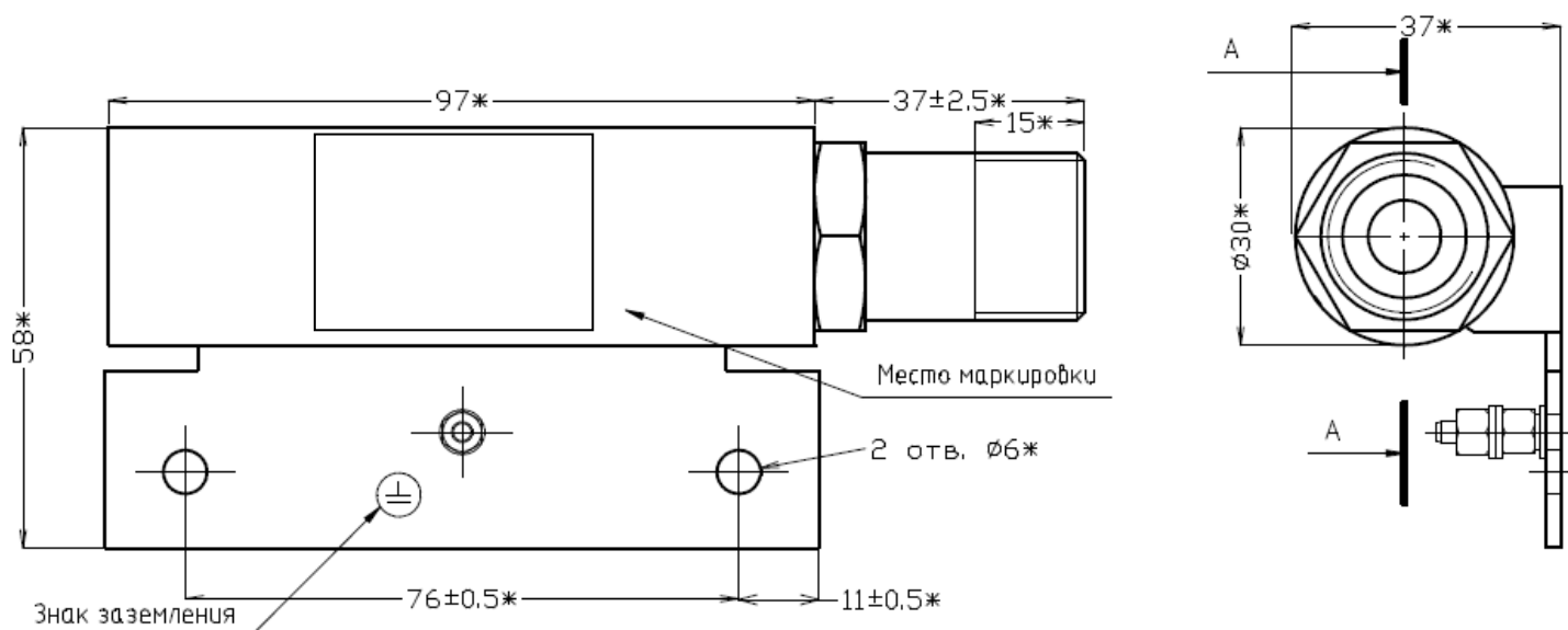
Рис.1 Габаритные и установочные размеры исполнительного блока Ex IO102 MK
