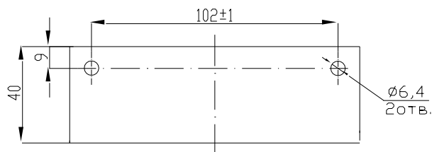
Блок магнита
