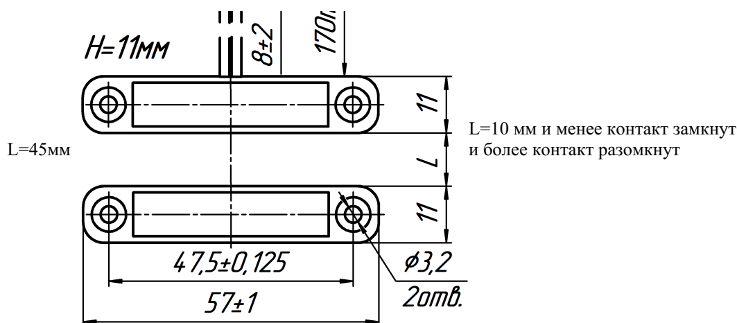
Рис.1. Габаритные и присоединительные размеры извещателя
