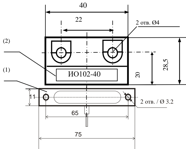
Рис.3 Габаритные размеры (1)- датчик; (2)- магнит
