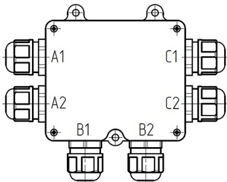
Схема 1 (вид спереди)
