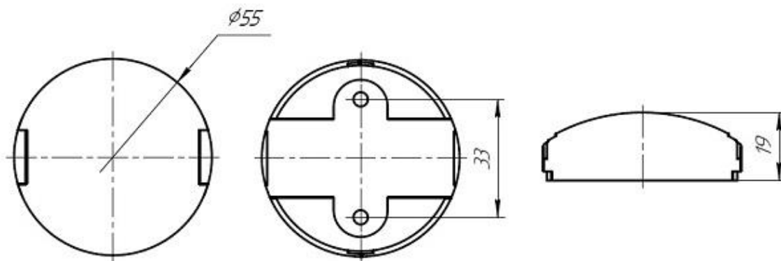
Габаритные и присоединительные размеры.
