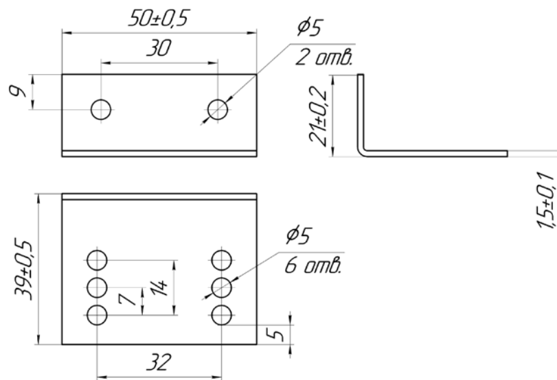
Рис.1. Габаритные и присоединительные размеры кронштейна К-20/50 АЯКС
